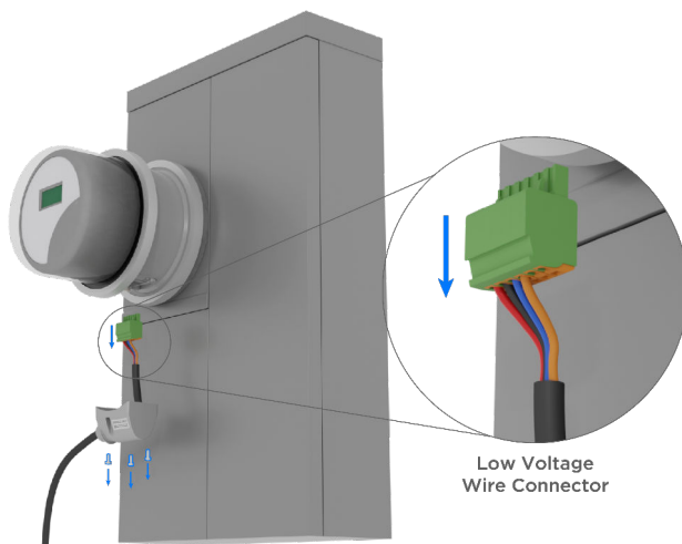
図 5. 低電圧ワイヤ コネクタ
