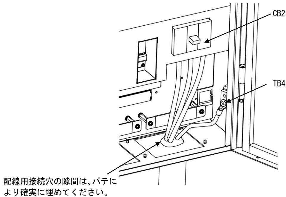
配線用接続穴のパテ埋め（系統出力側の例）
