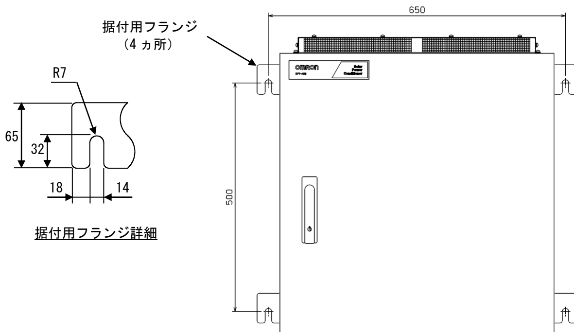
図 8-2 壁掛けの設置方法
