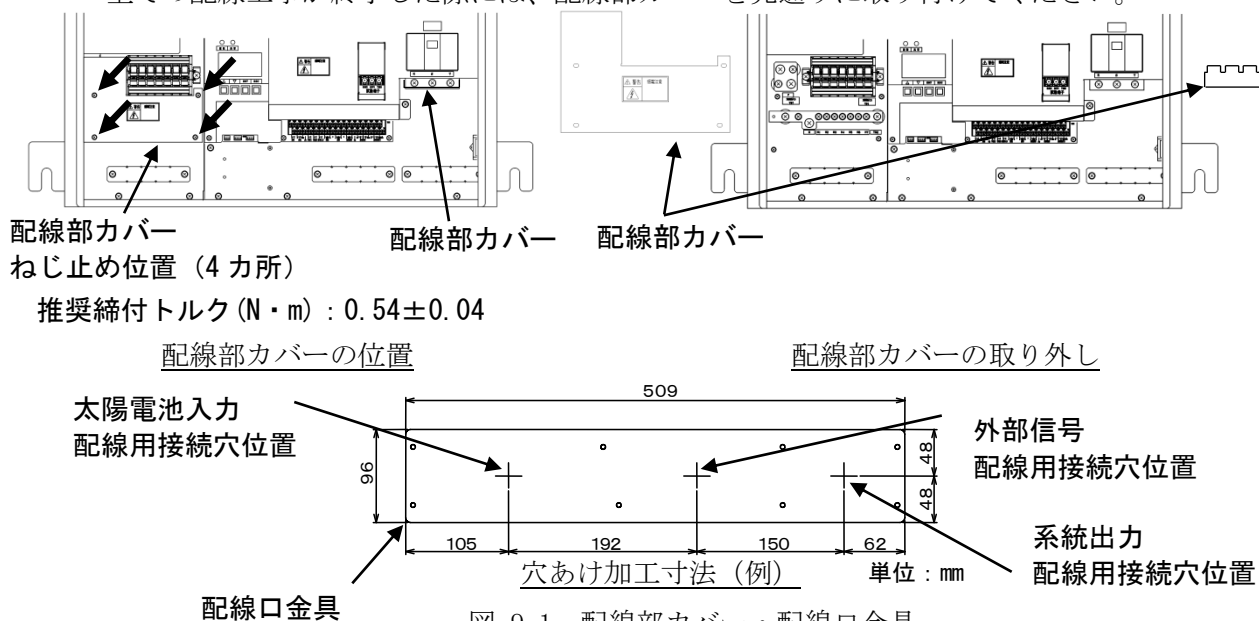
図 9-1 配線部カバー・配線口金具
