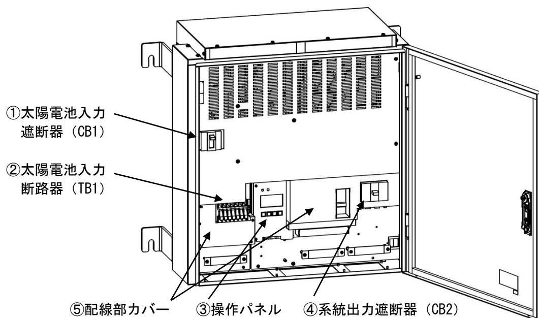
図 7-3 太陽光発電用パワーコンディショナの扉を開けた状態 (標準品)
