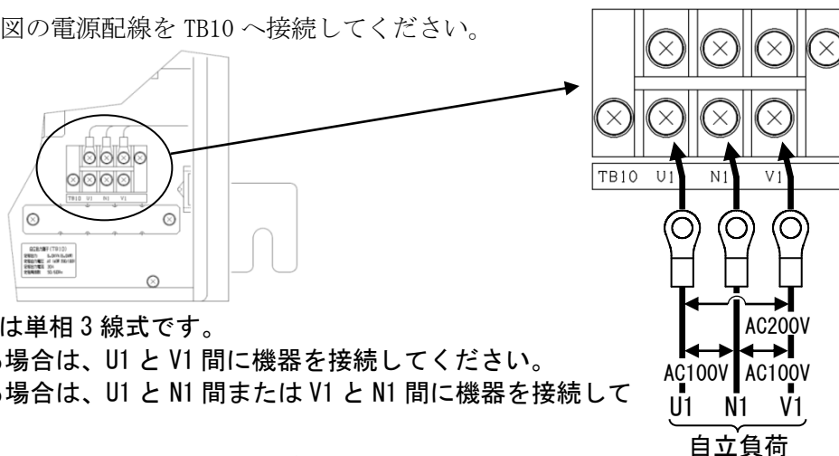
図 9-9 自立出力端子台接続図
