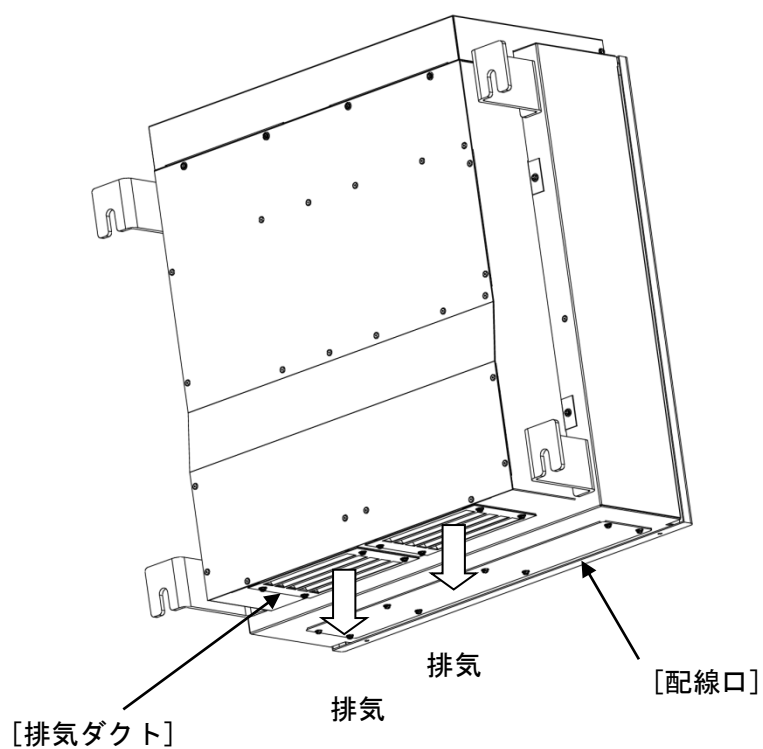
図 7-2 太陽光発電用パワーコンディショナ外観（裏面）
