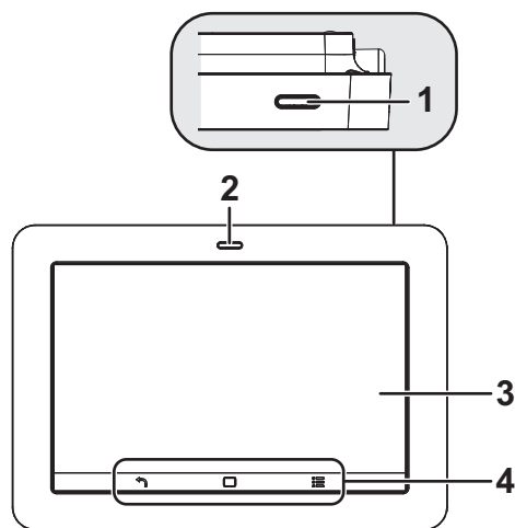
正面図
