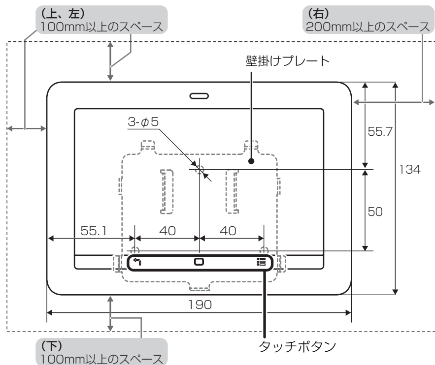
取り付け寸法図 (単位 : mm)
