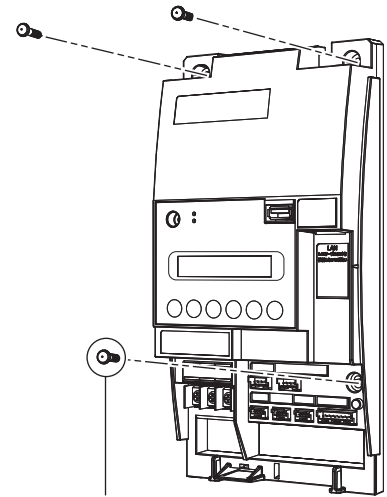
壁取り付け用木ねじ （ 4.1 \times 25 ）（同梱）
