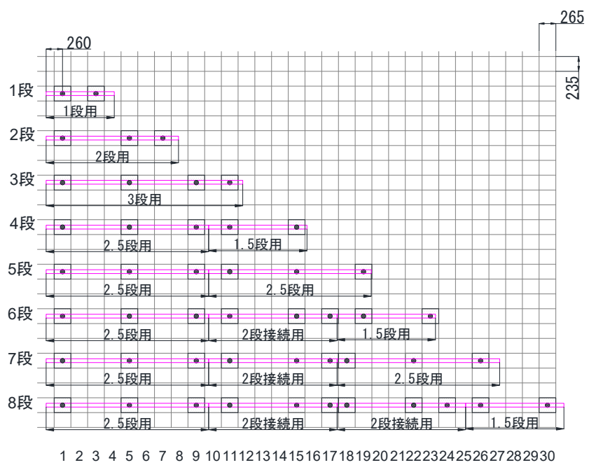
和瓦53Aの配置
