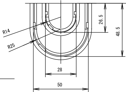
U字穴詳細 1 : 2
