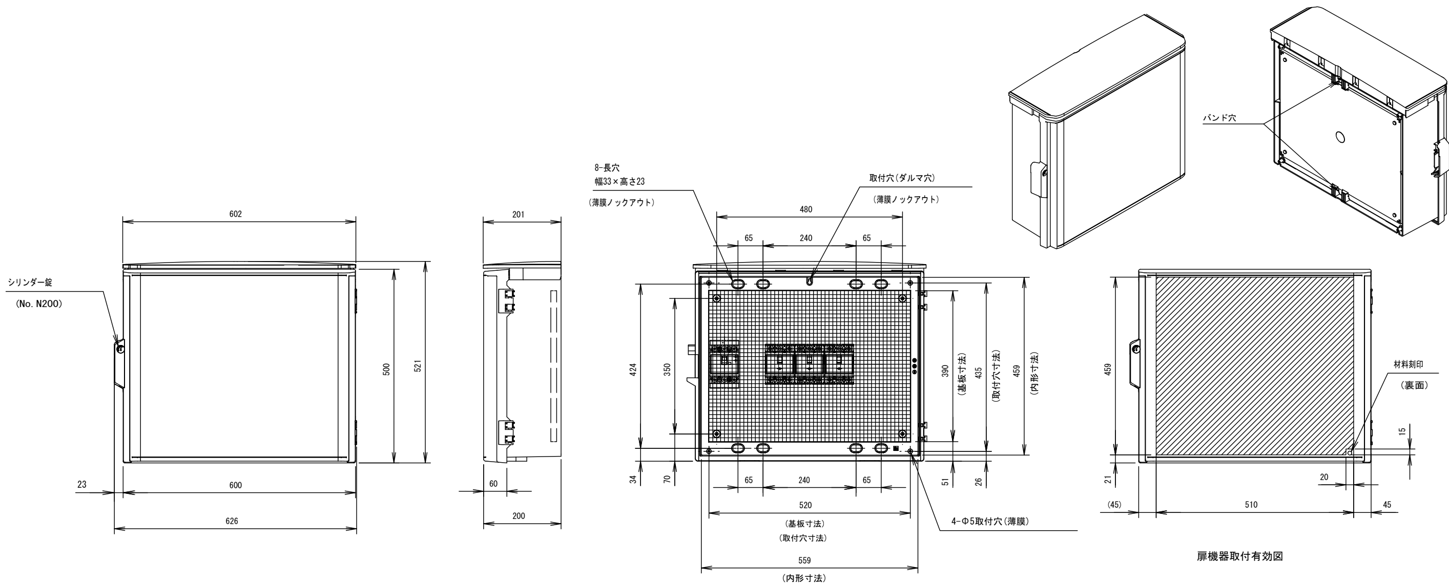
ボデー図
