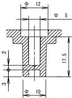
取付穴断面 1 : 1
