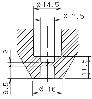
取付穴断面 1 : 1
