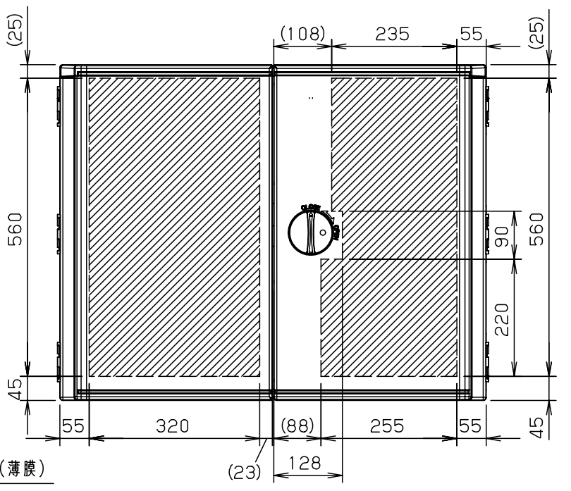
扉機器取付有効図
