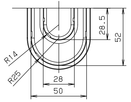
U字穴詳細 1 : 2
