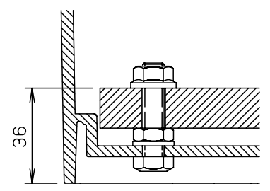
基板取付部詳細 1 : 2
